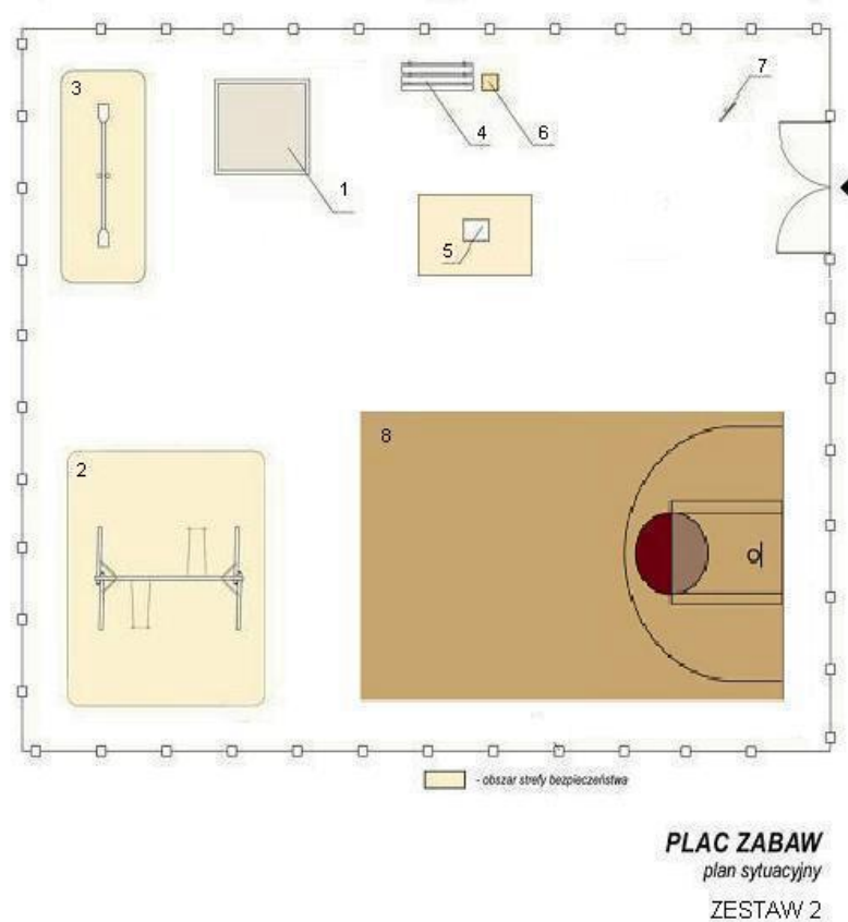
Plan sytuacyjny placu zabaw i rekreacji
